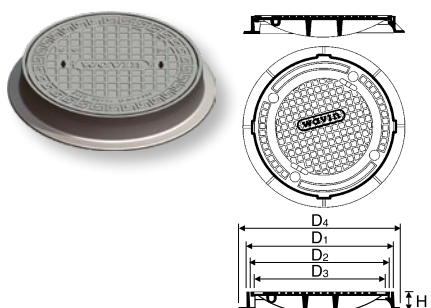
Litinový poklop
