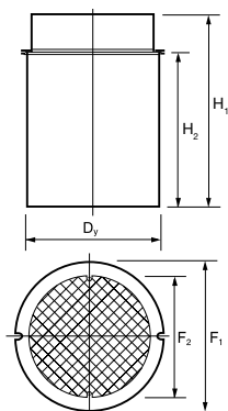
Litínový poklop 3 t – s teleskopickou rourou
