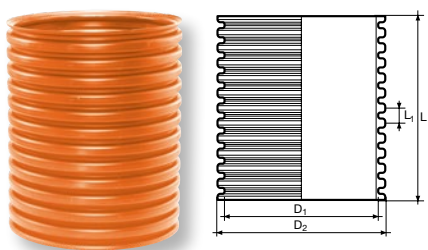
Šachtová vlnková roura SN4
