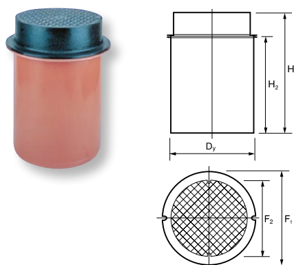
PVC poklop A15 – s teleskopickou rourou
