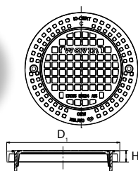
Litinový poklop A15 – do šachtové roury
