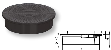
Plastový poklop A15 – do šachtové roury
