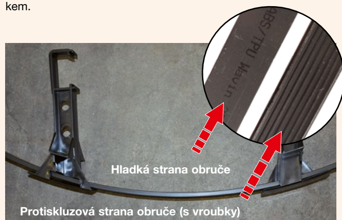
Umístění konzol žebříku na pásu
