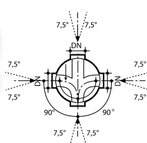
Šachtové dno Tegra 1000 NG – pro hladké potrubí (KG, KG 2000) sběrné dno pod úhlem 90° – typ X
