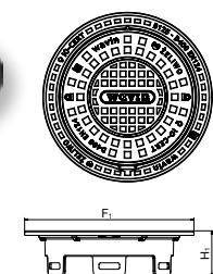
Litinový poklop B125 Ø 425 mm – kulatý do teleskopické roury
